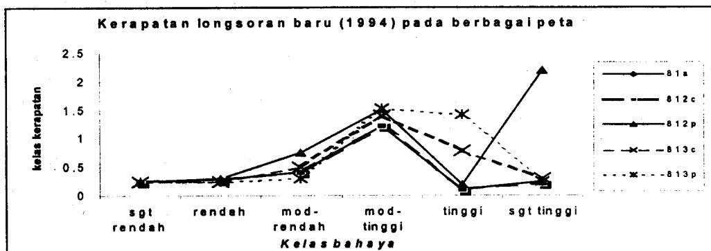
Gambar 5. Perbandingan hasil pemetaan tahun 1981 dengan cara berbeda yang diuji berdasarkan data longsor tahun 1994
