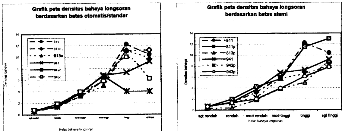
Gambar 4. Perbandingan hasil ketiga cara pemetaan dengan prosedur penarikan batas kelas (a) secara standar dan (b) berdasarkan pola data
